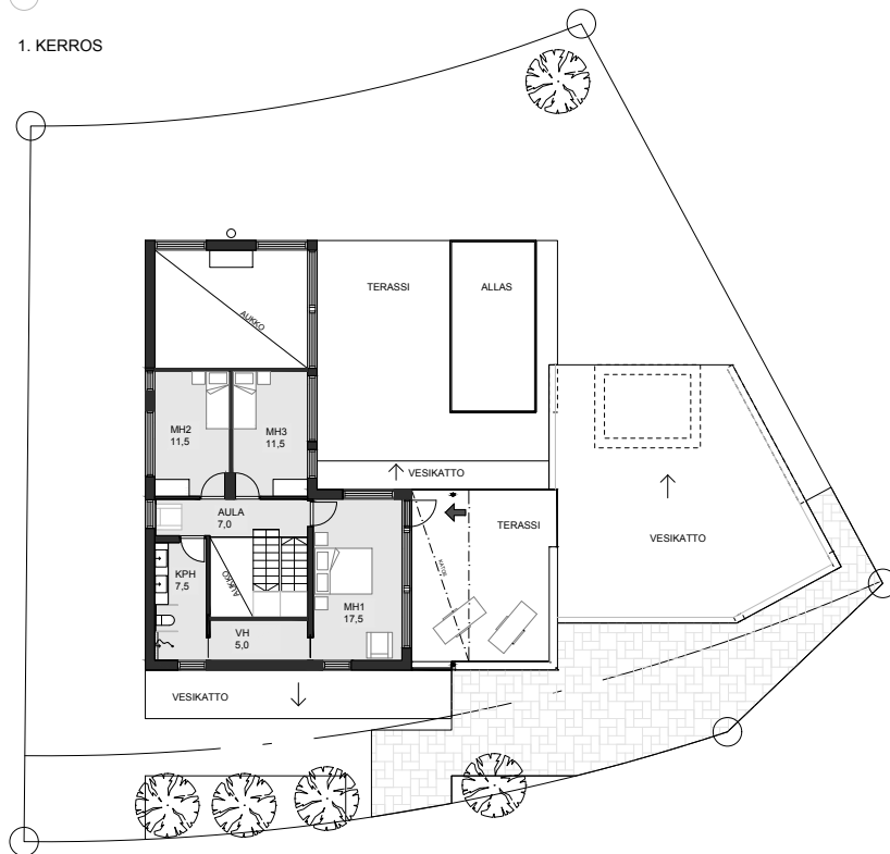
2. KERROS
